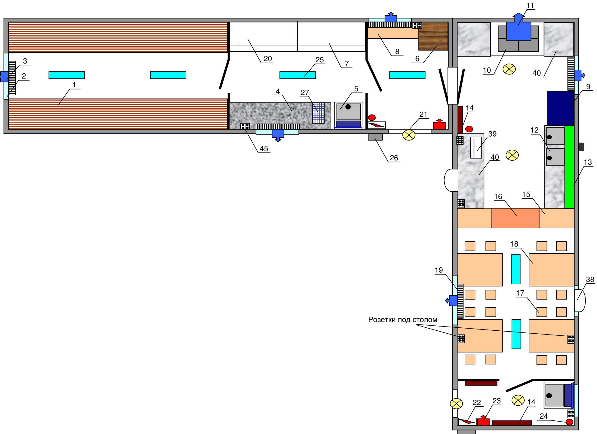
НМЗ "ЮПИТЕР -8.07" кухня-столовая на 16 человек со складом (2,8х10м)
