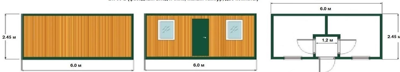
БК-05-2 (фасадный вход и окна, малый тамбур, две комнаты)
