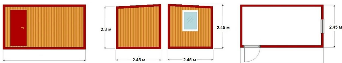
БС-04-4.5 (без тамбура, фасадный вход, торцевое окно)
