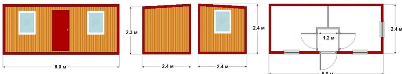
БС-05-2А (малый тамбур, две комнаты, три окна)
