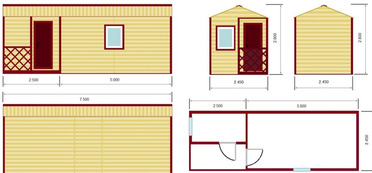
Планировка Вагон-дом "Дача-3" (2,45 x 7,50 x 2,40/2,80)
