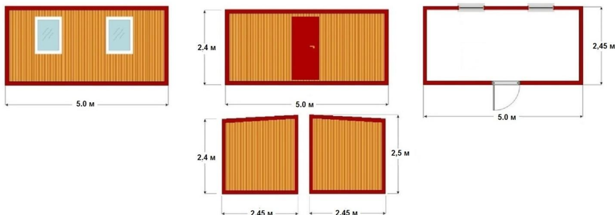
Вагон-дом "Дачник-1" тип ВД-06МУ-5.0 (без тамбура, два окна)
