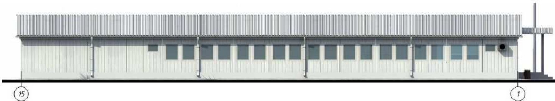
Фасад 15-1
